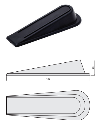
Door Stop WEDGE
