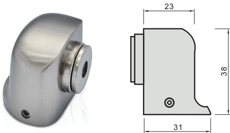
Door Stop KHAN
