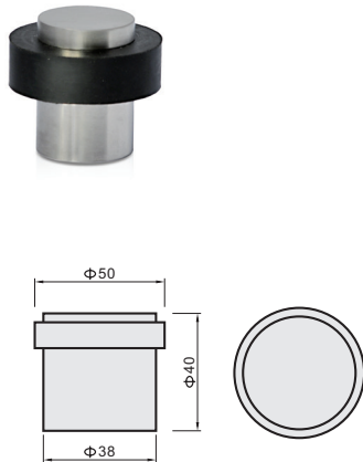
Door Stop BANKS
