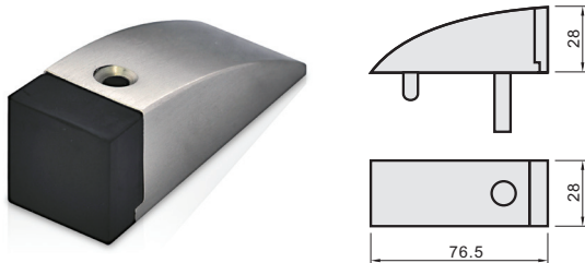
Door Stop DESAR
